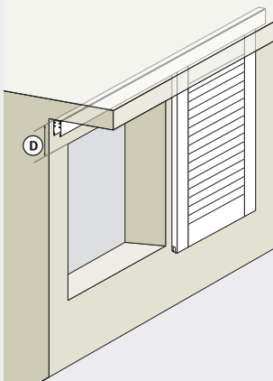
Guidage haut sous dalle
