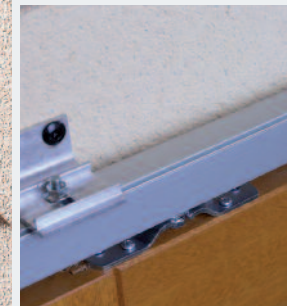
Rail (capot non monté)
