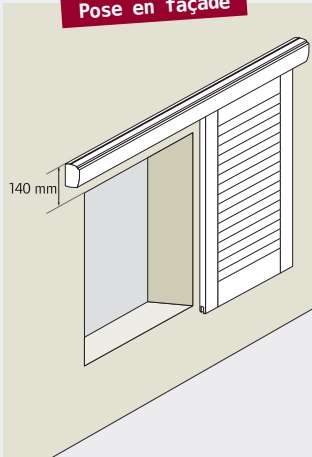
Guidage haut en façade
